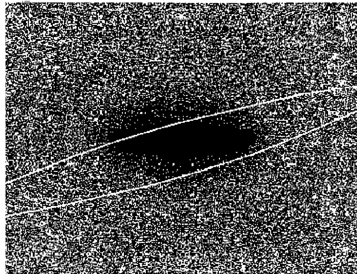
focalizzazione dovuta all'azione della massa negativa
