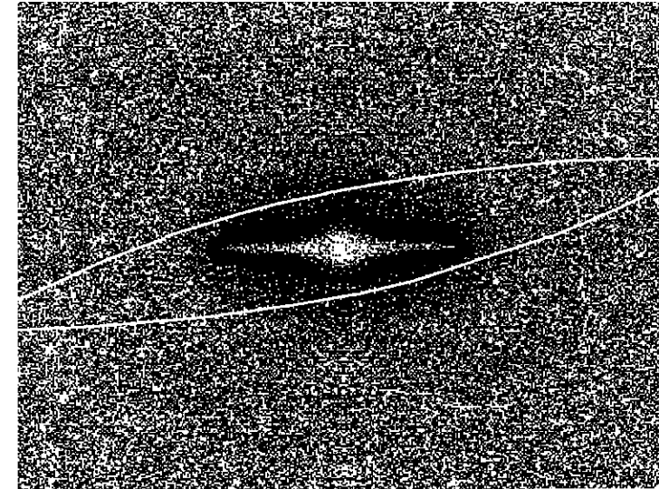
i due effetti, combinati
