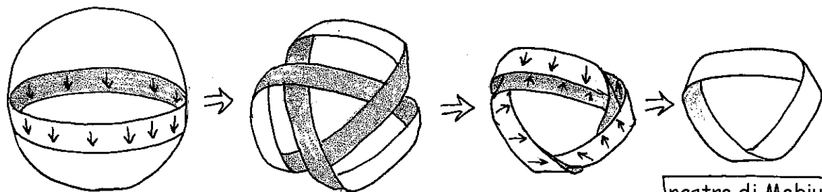
vicinanze dell'equatore di questa sfera spazio-tempo
