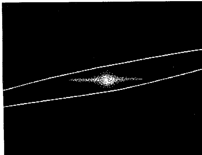
effetto di lente gravitazionale, galassia isolata
