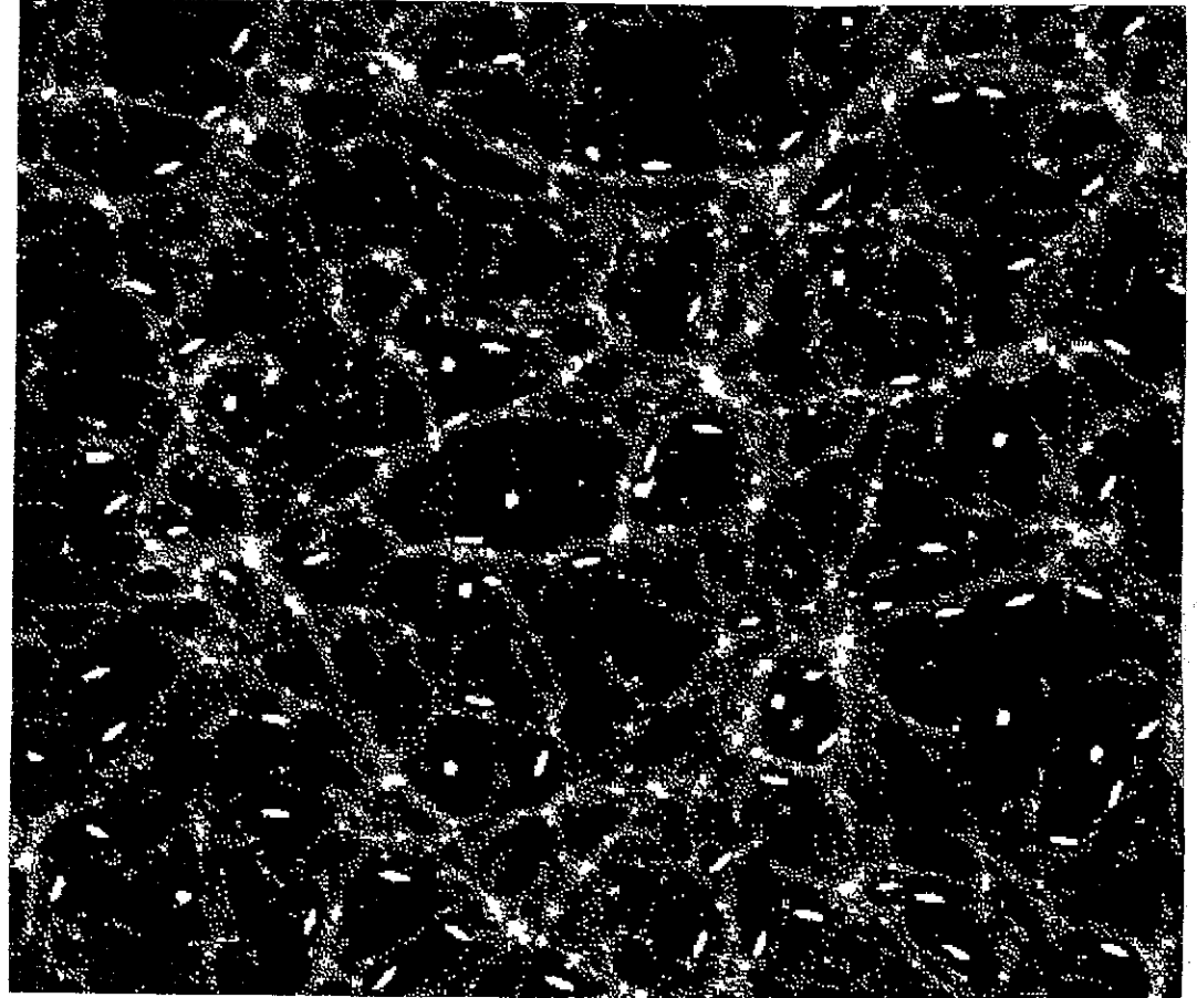
La prima mappa della MATERIA OSCURA pubblicata nel 2000
