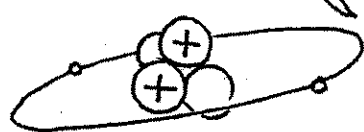
Noyau d'hélium
